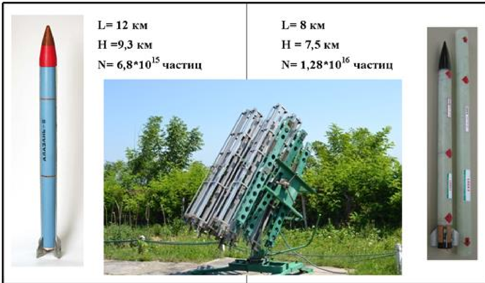
Расми 2. Дастгоҳи мушакандози ТКБ040К-01 ва мушаки зидди жолаи Кристалл
