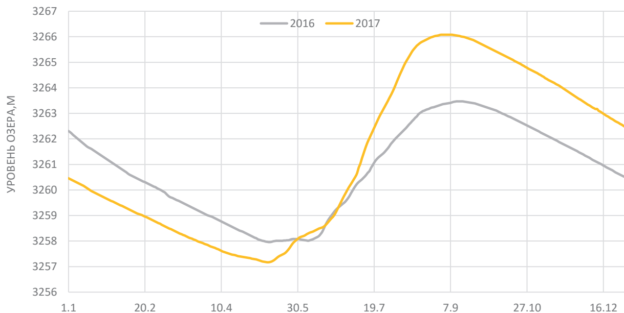
Сатҳи оби кули Сарез (солҳои 2016–2017) Уровень воды озера Сарез (2016–2017)
