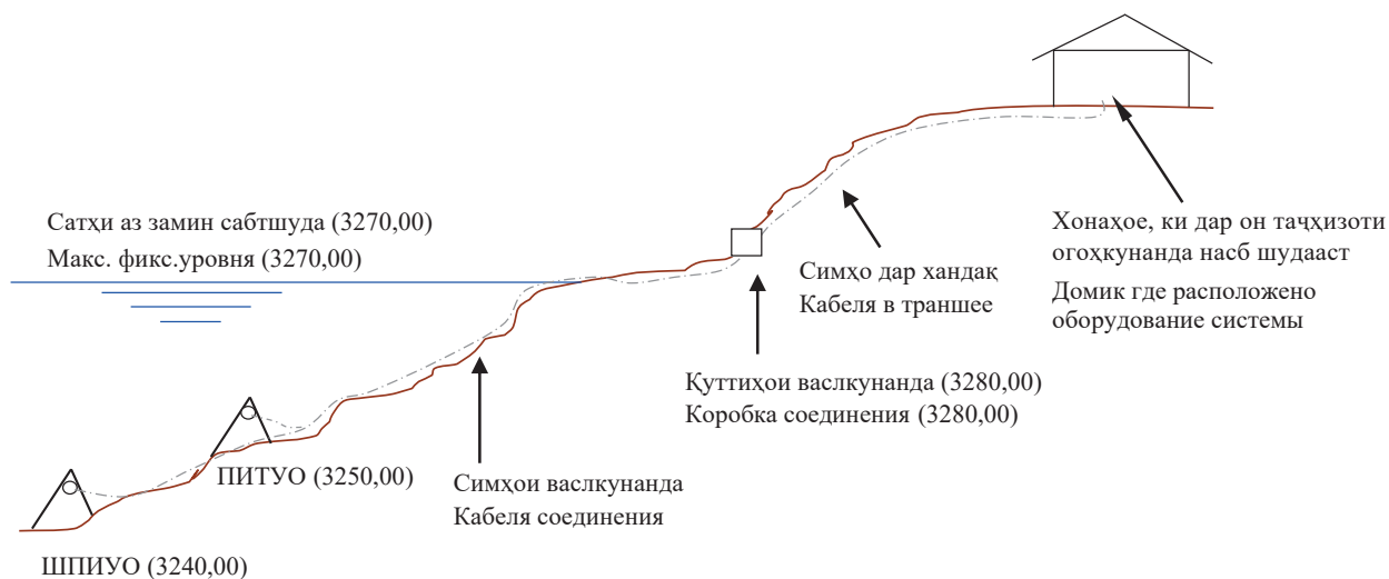
Таҷҳизотҳо барои ченкунии сатҳи оби дарёи Мурғоб, ки аз кули Сарез ҷорӣ мешавад Оборудования для измерения уровня воды реки Мургаб, протекающая из озера Сарез
