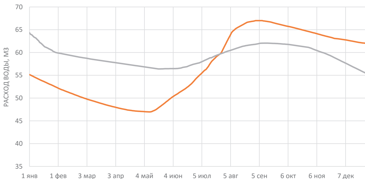
Ихроҷи дарёи Мурғоб (солҳои 2016–2017) Расход воды река Мургаб (2016–2017)
